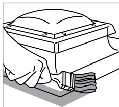
Tætning ved ovenlyskupler.
